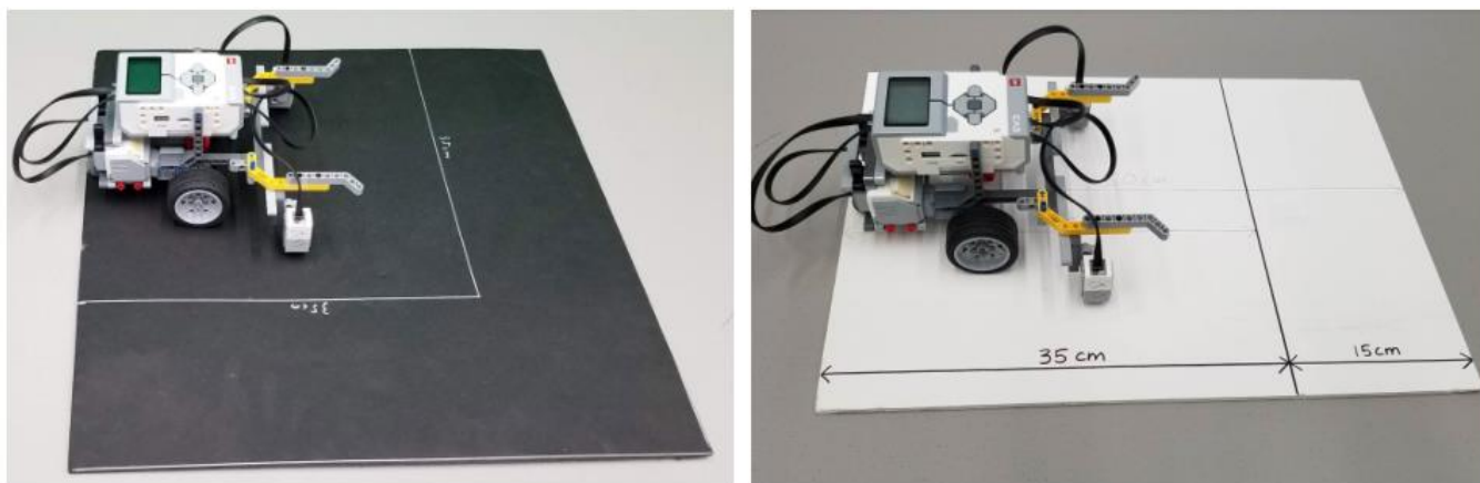
图 3 如何检查机器人的宽度和长度。
